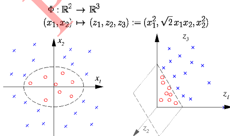
Hình 5.21. Ví dụ một ánh xạ từ không gian hai chiều sang không gian ba chiều. Trong không gian mới, các ví dụ có thể phân chia tuyến tính bởi một mặt phẳng.
