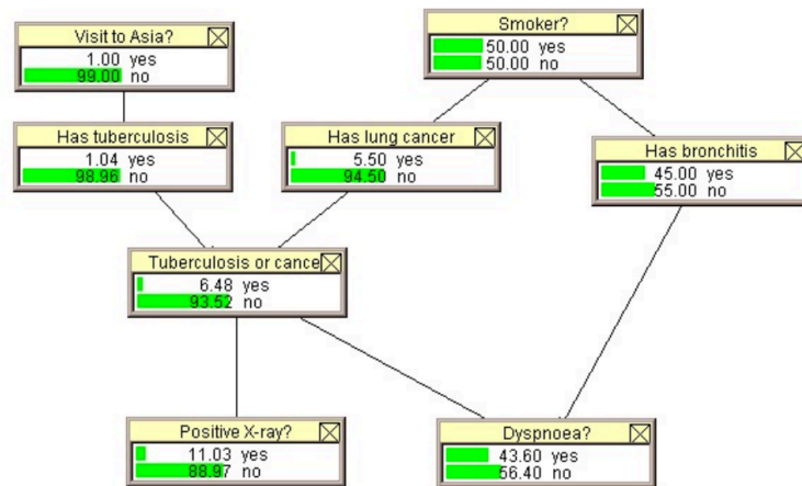
Hình 4.20. Mạng Bayes chẩn đoán bệnh hô hấp
